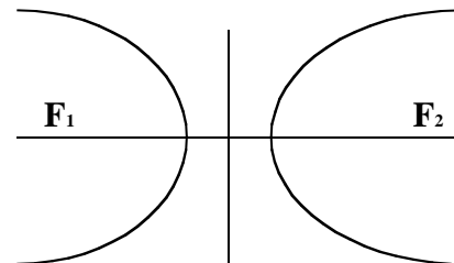
HIPERBOLA
